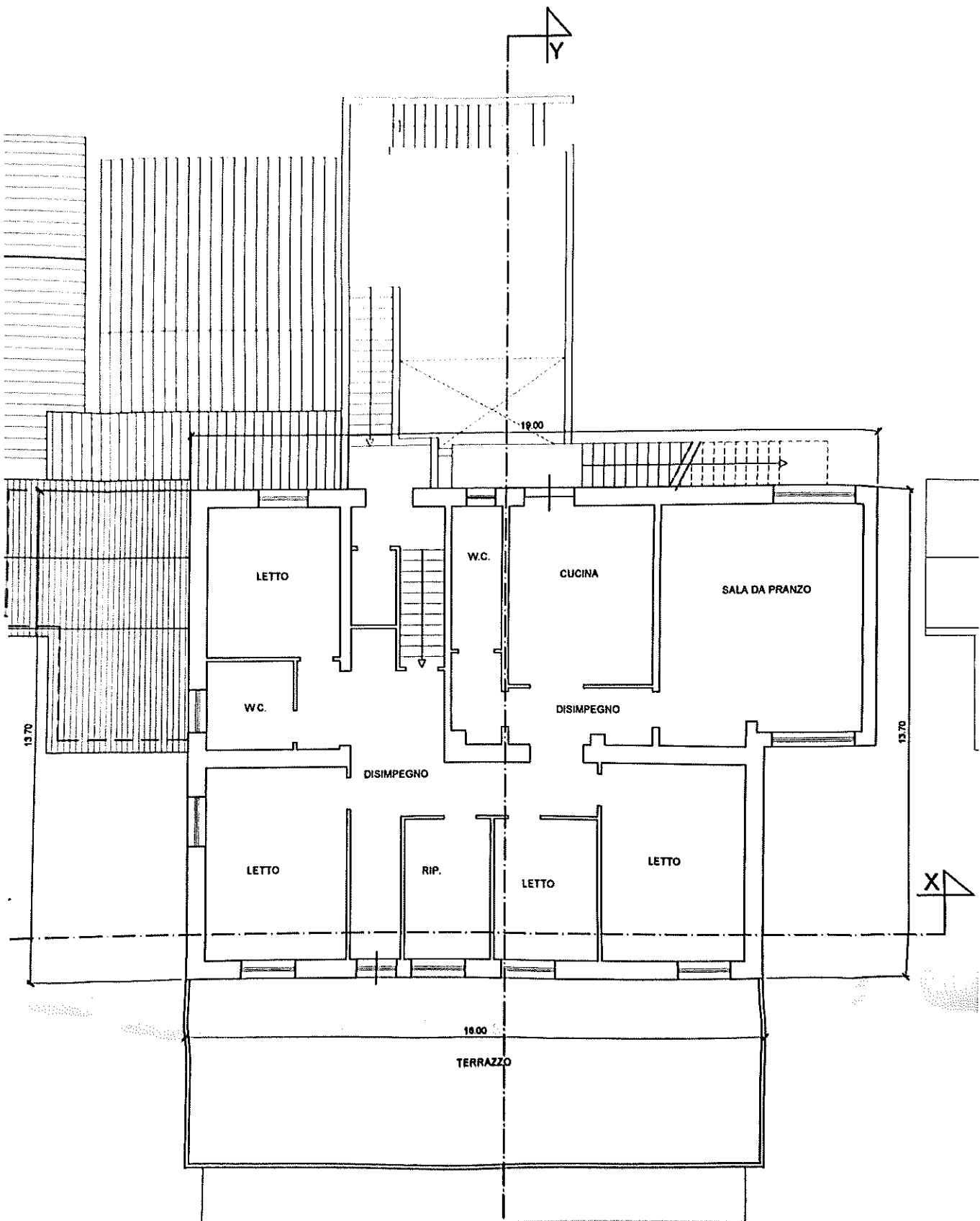
PIANTA PIANO SECONDO H. ml 3.00 NON OGGETTO D'INTERVENTO
